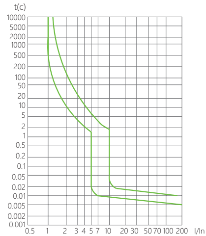
Характеристика С
